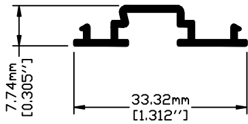
Clave: 9075 Tapa Bolsa Perimetro Anodizable: 11.54 cm
