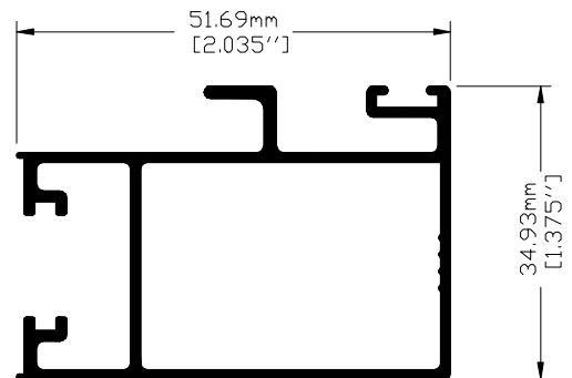
Clave: 7848 / L7848 Traslape Puerta Perimetro Anodizable: 26.21 cm
