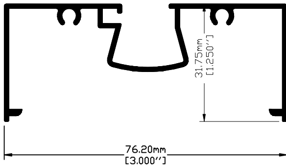
Clave: 10235 Bolsa Corta Perimetro Anodizable: 40.86 cm
