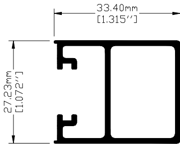
Clave: 7843 Cerco Ventana Perimetro Anodizable: 19.00 cm
