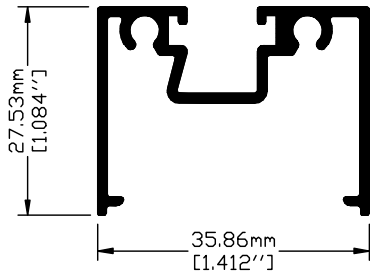
Clave: 9073 Bolsa Perimetro Anodizable: 25.98 cm
