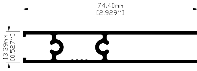
Clave: 7825 / L7825 Zoclo Puerta Perimetro Anodizable: 29.71 cm
