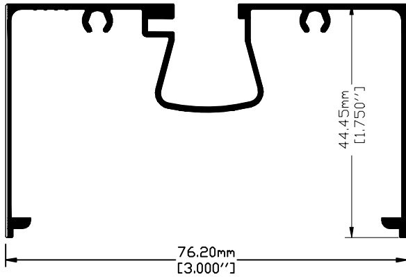
Clave: 9135 / L9135 Bolsa Perimetro Anodizable: 46.57 cm
