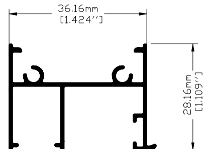
Clave: 15309 Jamba Cabezal Perimetro Anodizable: 10.92 cm
