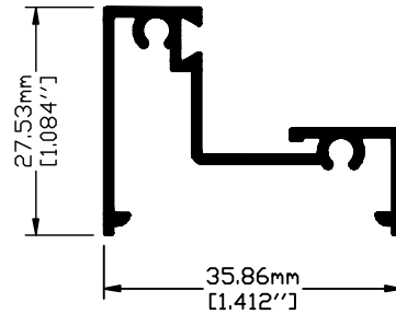
Clave: 9074 Escalonado Perimetro Anodizable: 22.66 cm
