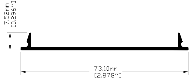
Clave: 7316 Tapa Lisa Perimetro Anodizable: 17.25 cm
