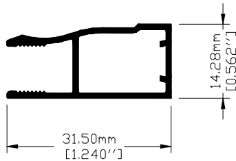
Clave: 11035 Marco de 1 1/4" Perimetro Anodizable: 18.18 cm
