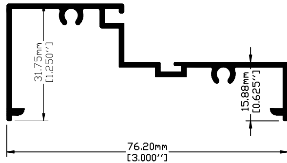
Clave: 10236 Escalonado Corto Perimetro Anodizable: 34.62 cm
