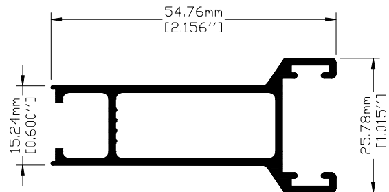
Clave: 7822 Cerco OXO Perimetro Anodizable: 22.18 cm
