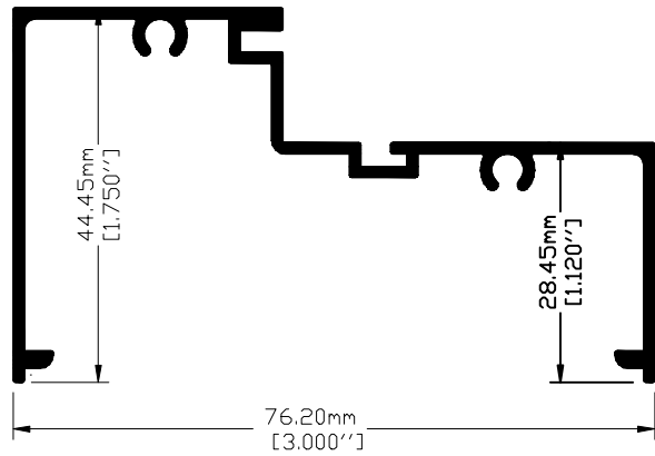
Clave: 9136 / L9136 Escalonado Perimetro Anodizable: 39.43 cm
