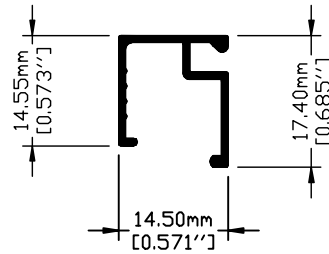
Clave: 6370 Junquillo Perimetro Anodizable: 10.84 cm
