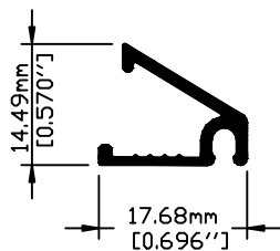
Clave: L6371 Junquillo Biselado Perimetro Anodizable: 08.13 cm
