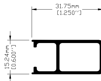
Clave: 8320 Cerco Ventana Perimetro Anodizable: 11.97 cm
