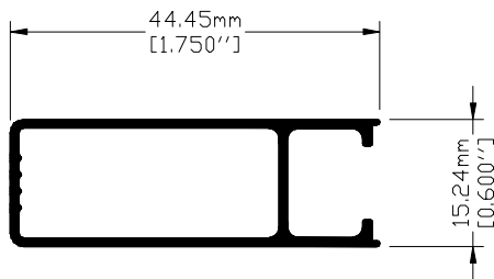
Clave: 7821 / L7821 Cerco Puerta Perimetro Anodizable: 14.51 cm
