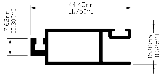
Clave: 6534 Cerco Mosquitero Perimetro Anodizable: 17.44 cm
