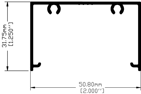
Clave: 8591 / L8591 Bolsa Lisa Perimetro Anodizable: 27.39 cm
